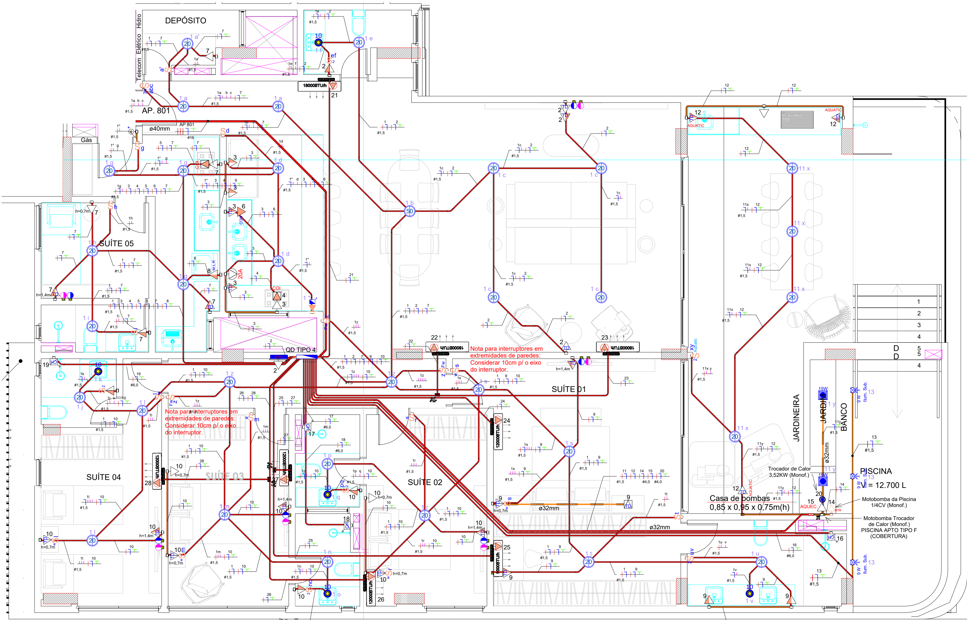
1 APTO TIPO F 1 : 50
